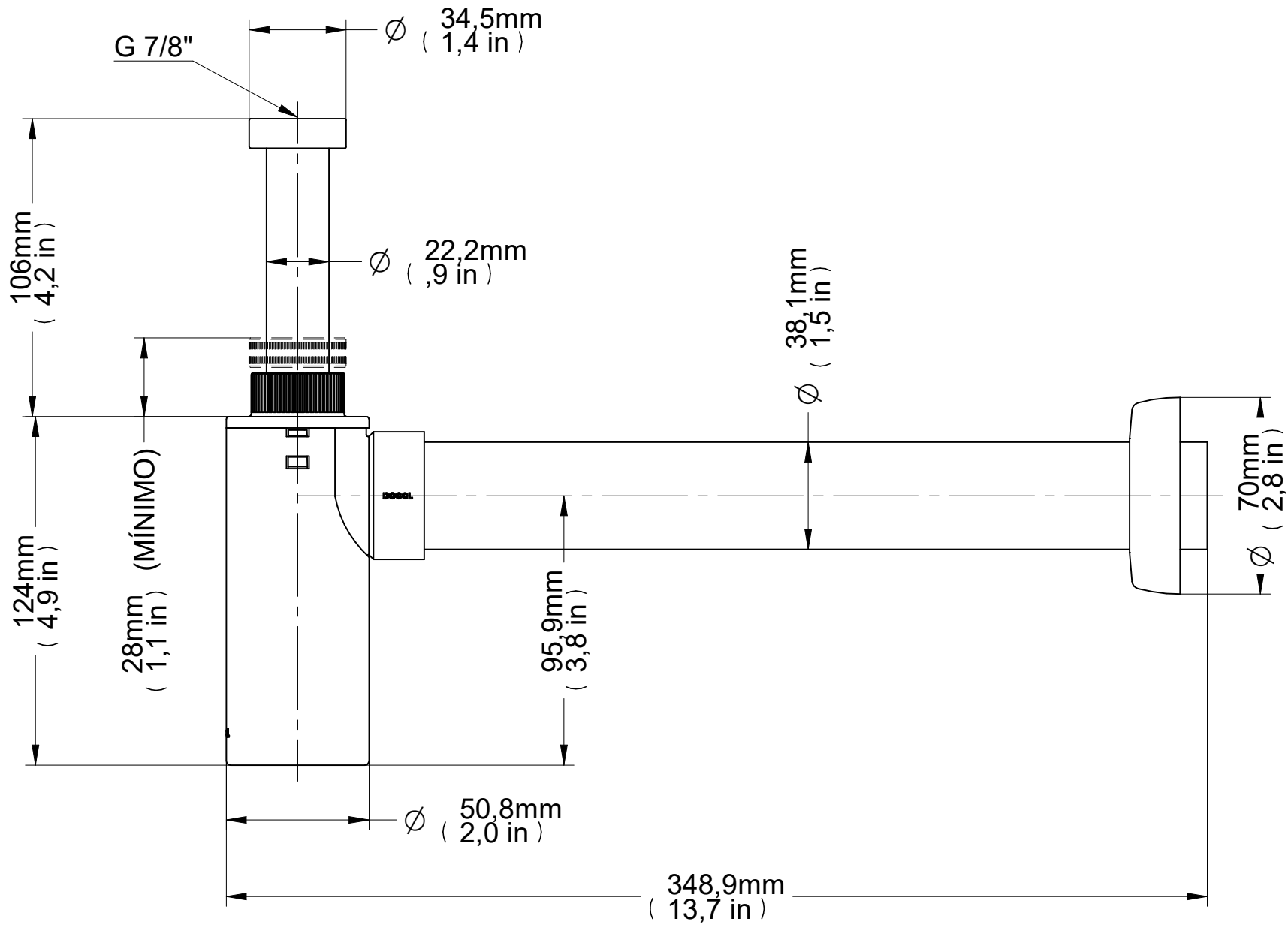
SIFAO PARA LAVATORIO - BITOLA 1" X 1.1/2" LAVATORY TRAP - 1"X1.1/2" SIFON - 1"X1.1/2"
