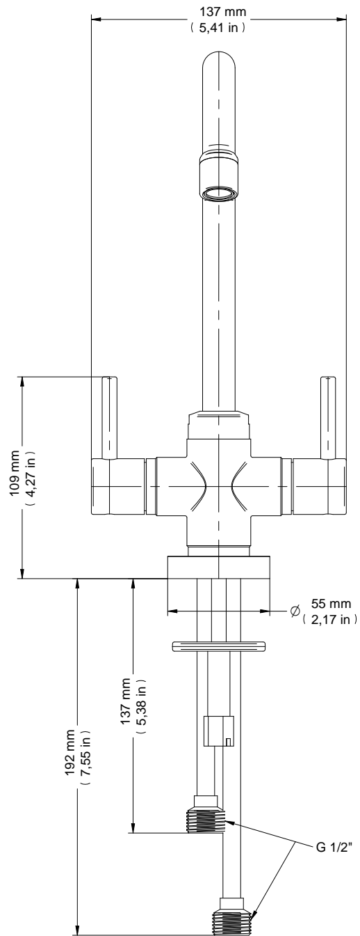
MISTURADOR MONOBLOCO COZINHA/LAVATORIO UNO - CHROME SINGLE-HOLE KITCHEN/LAV FAUCET - 1/2" - UNO MEZCLADOR MONOBLOCK DE MESA - COCINA Y LAVATORIO - 1/2" - UNO
