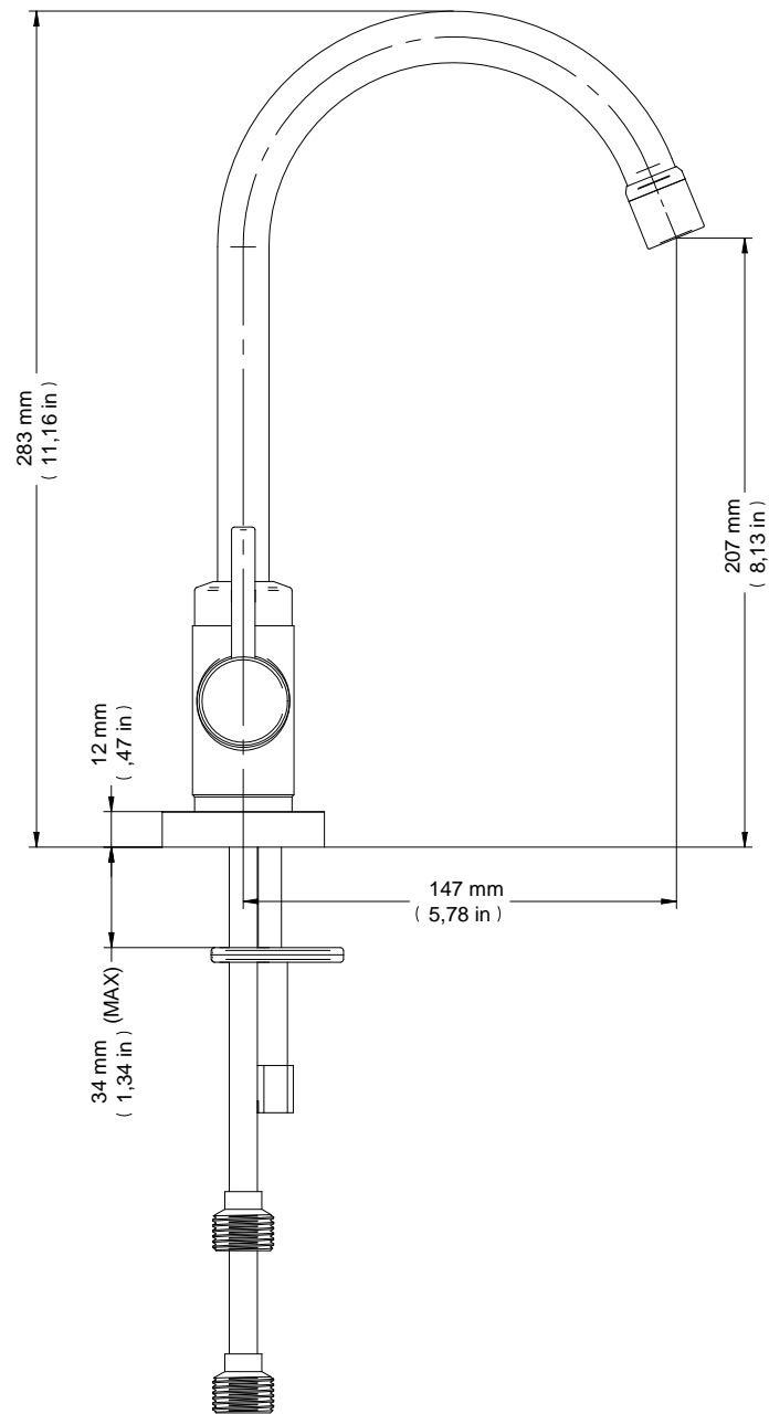
MISTURADOR MONOBLOCO COZINHA/LAVATORIO UNO - CHROME SINGLE-HOLE KITCHEN/LAV FAUCET - 1/2" - UNO MEZCLADOR MONOBLOCK DE MESA - COCINA Y LAVATORIO - 1/2" - UNO
