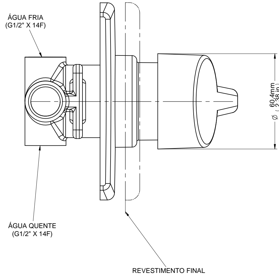
ACABAMENTO MISTURADOR MONOCOMANDO CHUVEIRO 1/2 NEXUS SINGLE CONTROL SHOWER TRIM (WITHOUT VALVE) - 1/2" - NEXUS ACABADO MONOCOMANDO DUCHA - 1/2" - NEXUS
