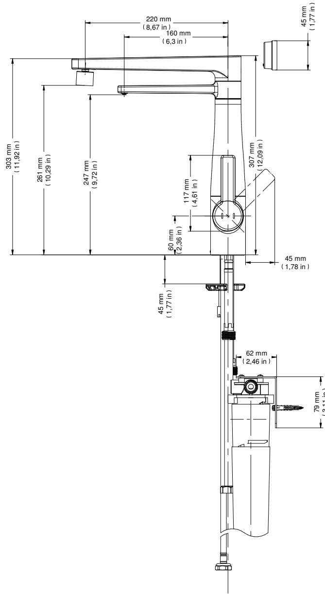
MISTURADOR MONOCOMANDO COZINHA C/ PURIFICADOR DE AGUA DOCOLVITALIS-CHROME SINGLE LEVER KITCHEN FAUCET WITH WATER PURIFIER DOCOLVITALIS-CHROME MEZCLADOR MONOCOMANDO COCINA CON PURIFICADOR DE AGUA DOCOLVITALIS-CHROME
